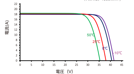
異なる温度下での I-V カーブ (AM1.5, 1000W/m 2 )
