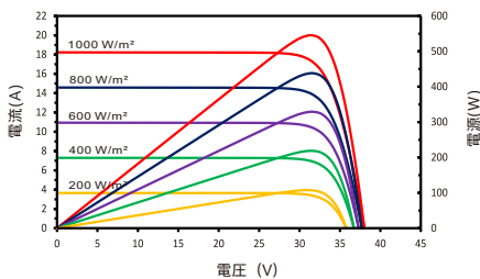
RSM110-8-545M 異なる照射量下での I-V カーブ
